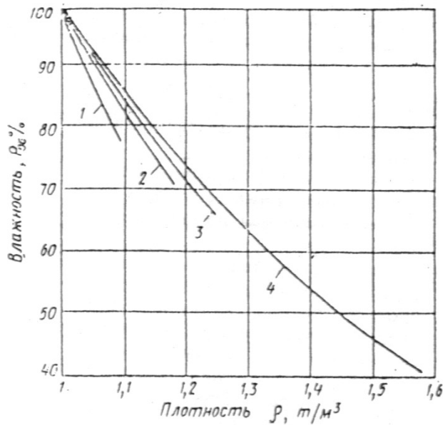
Рис. 5. Значения плотности в зависимости от влажности осадка станции осветления и обезжелезивания воды
